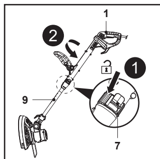
Fig. 9B (poziția inițială la 180°)
