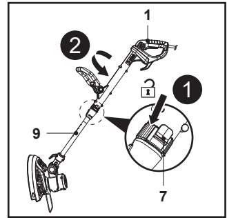
Fig. 9 B (posición inicial a 180°)
