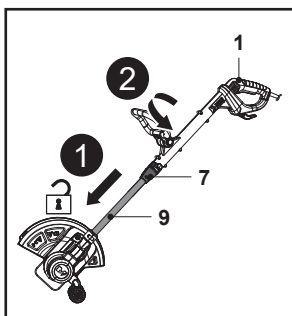
Fig. 9A (poziția inițială la 90°)
