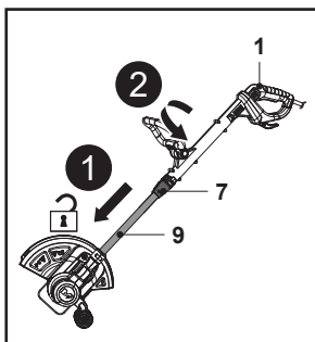
Fig. 9 A (posição inicial de 90°)
