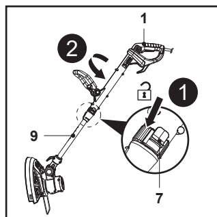
Fig. 9B (position initiale 180°)
