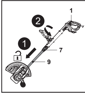
Şek. 9 A (ilk konum 90°)
