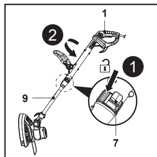
Rys. 9 B (położenie początkowe 180°)
