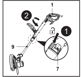
Şek. 9 B (ilk konum 180°)
