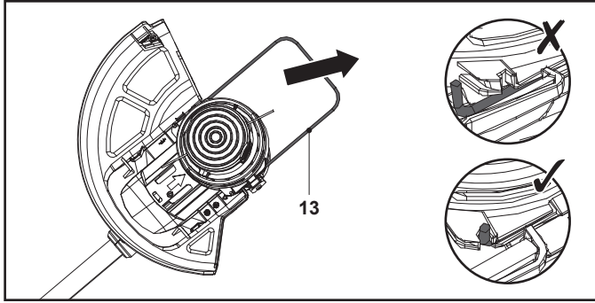
Şek. 12, budama / kenar kesme konumu
