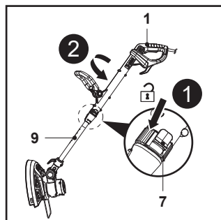
Fig. 9 B (posição inicial de 180°)
