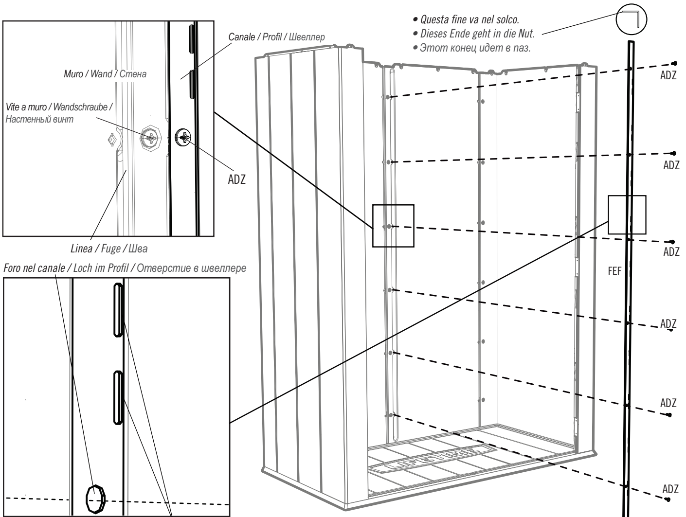
Fessure sul bordo destro del canale / Schlitze auf der rechten Kante des Profils / Прорезы на правом краю швеллера
