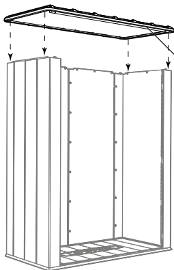
Parte anteriore del tetto / Vorderseite des Daches / Передняя часть крыши
