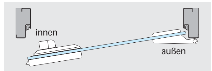
Bedienknebel auf Klemmplatenseite (DIN rechts auswärts)
