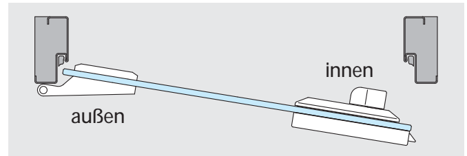
Bedienknebel auf Klemmplatenseite (DIN links auswärts)
