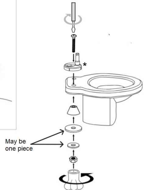
Bottom Fix
