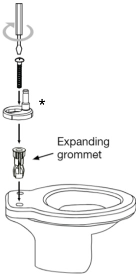
Top Fix
