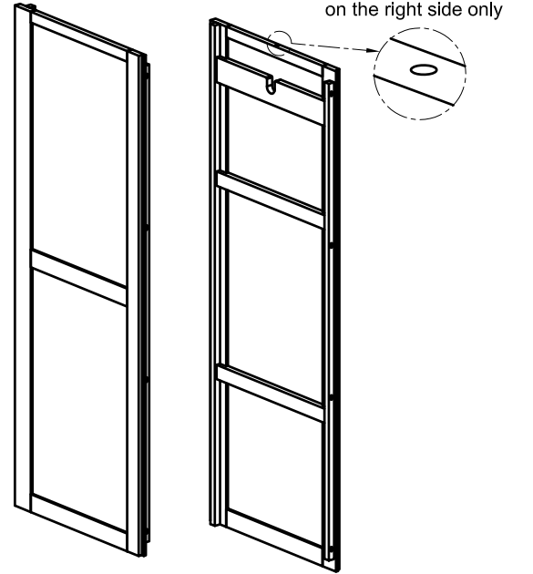
Ⓑ - RIGHT FRAME 1X LEFT FRAME 1X
