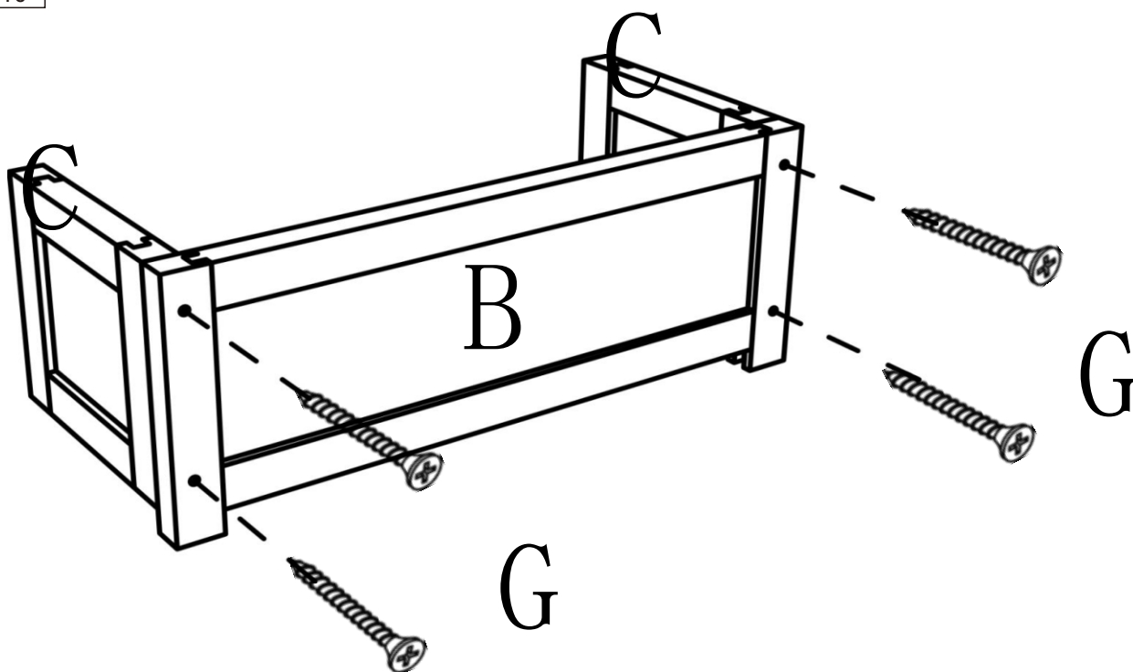
G x04 M4*40
