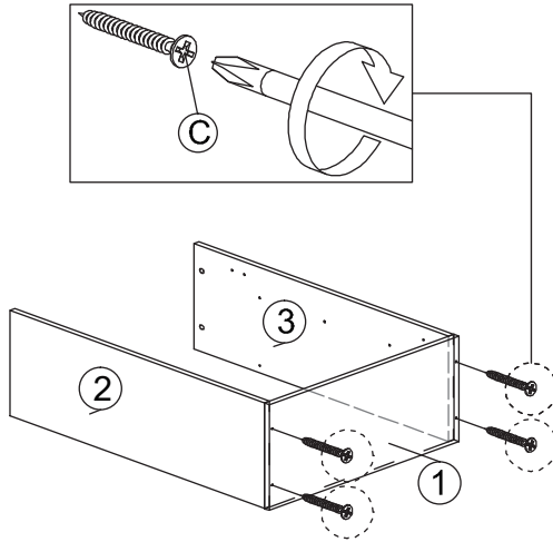
BOTTOM VIEW /VUE DE DESSOUS
