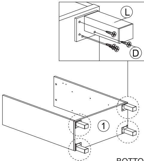
BOTTOM VIEW /VUE DE DESSOUS
