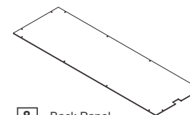
8 Back Panel (74.3(w)cmx23.5 (d)cm)
